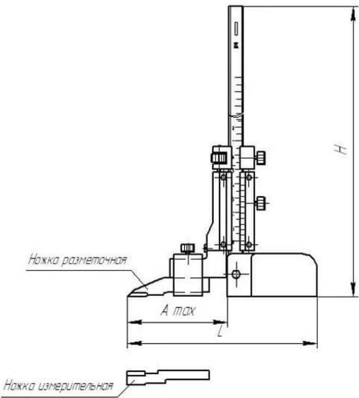
Штангенрейсмас ШР 250
