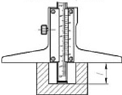
Схема измерения
